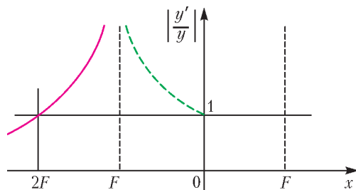
Рис. 2. Увеличение в линзе в зависимости от положения объекта слева от нее
