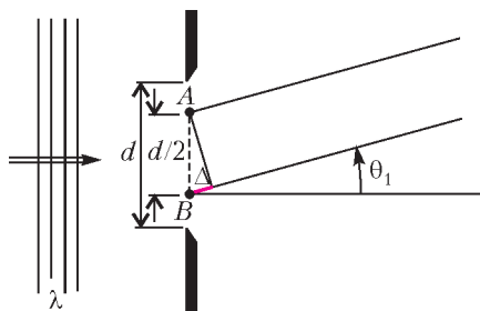
Рис. 4. Щель в плоском экране и направления, в которых волна, прошедшая через щель, гасит сама себя
